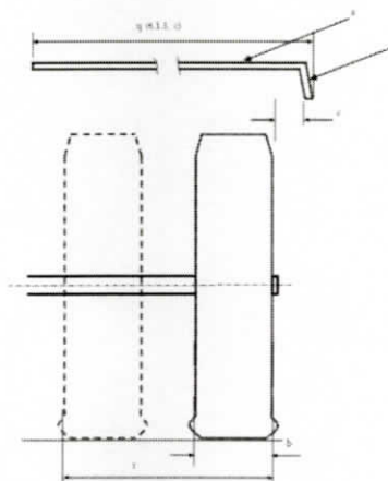
Figura N° 2, Anchura del guardabarros
